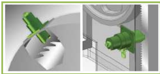
Buse spécifique 3 voies pour scie circulaire et ruban.
